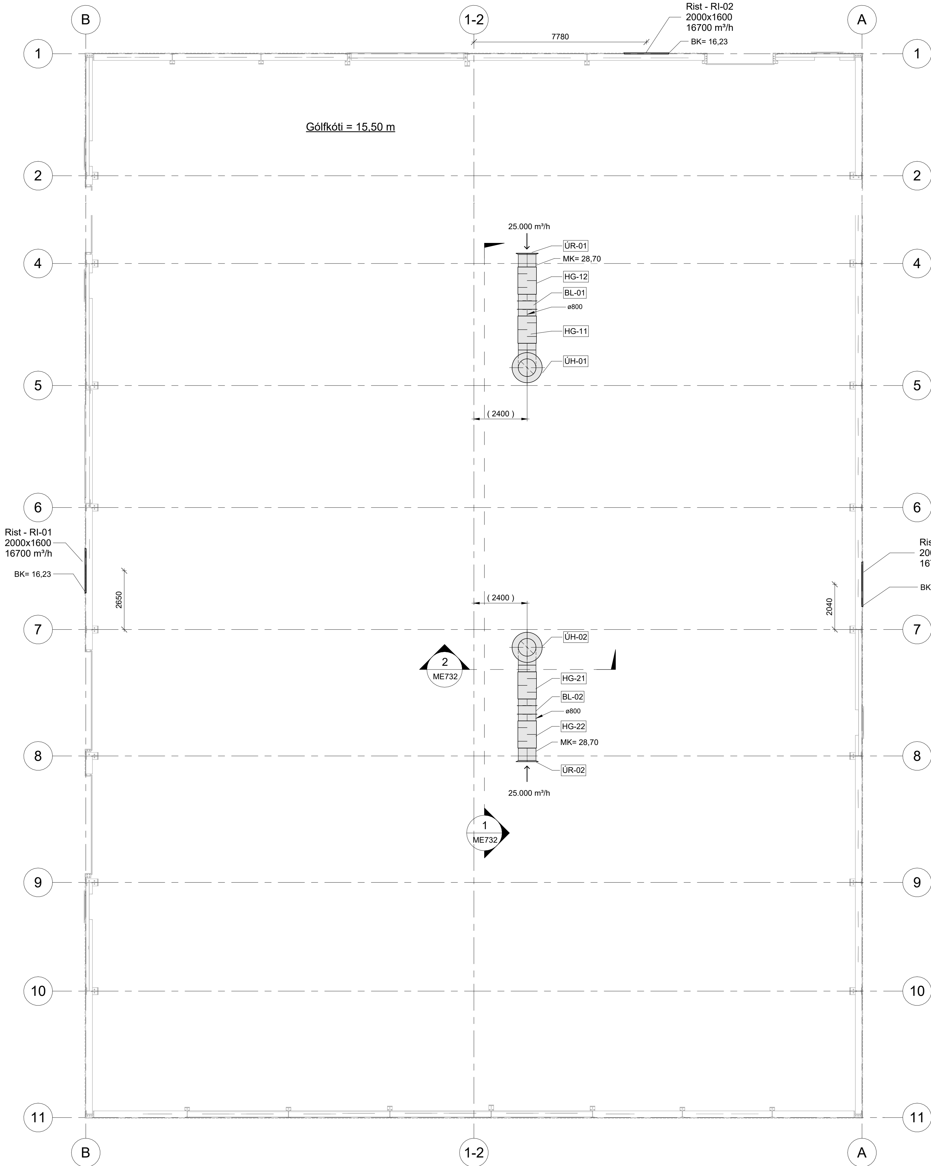
Grunnmynd 1 : 100
